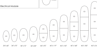
Electrical Module
